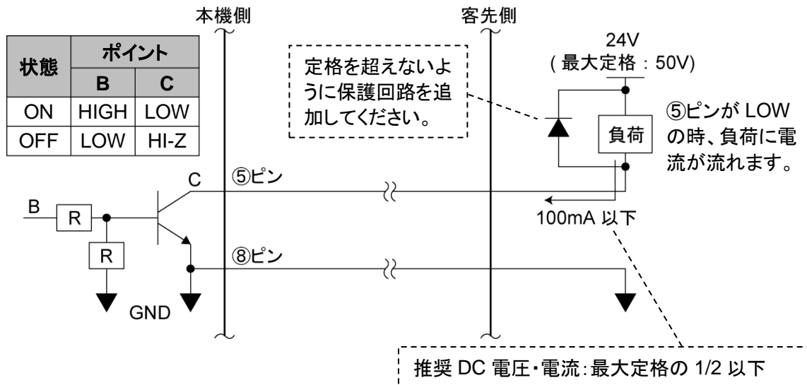
参考回路
