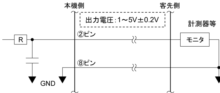
参考回路
